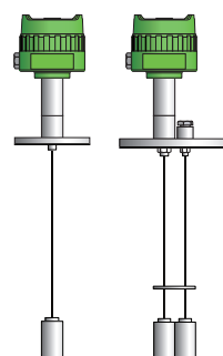
带接地线的探线 (Teflon)
